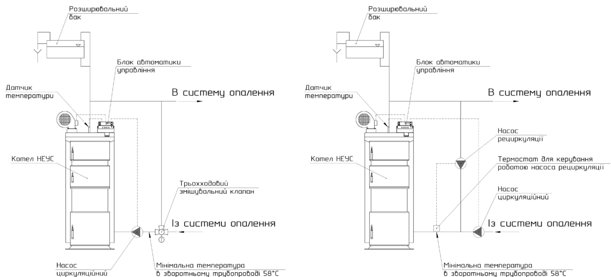
Рисунок 3 – Схеми підключення котла до системи опалення
