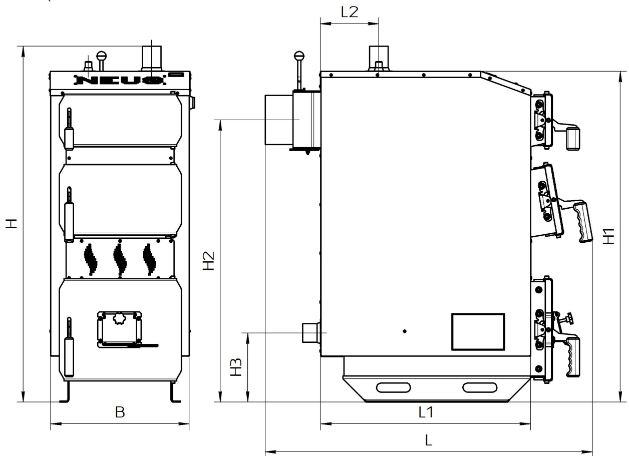
Рисунок 1 – Габаритне креслення котла Неус-Практик-М
