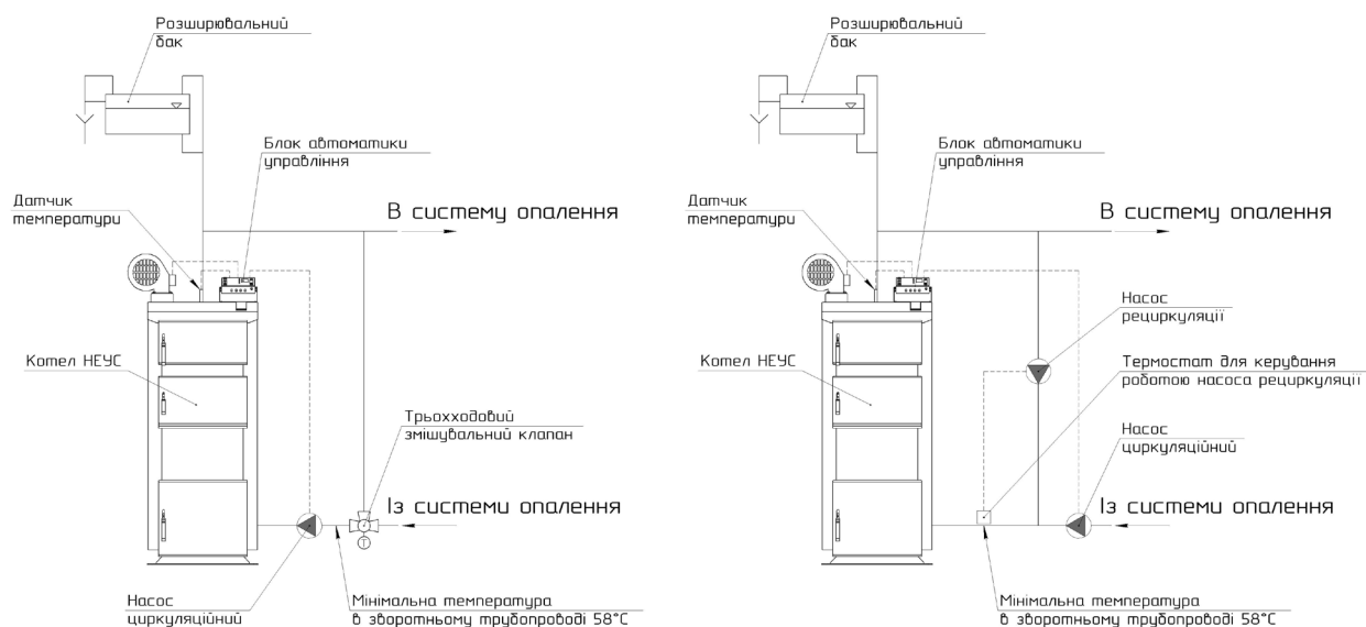
Рисунок 3 – Схеми підключення котла до системи опалення
